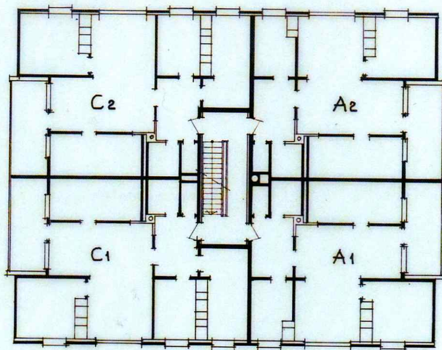
2., 3. OG 4. ETASJE
